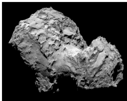
チュリュモワ-ゲラシメンコ彗星
